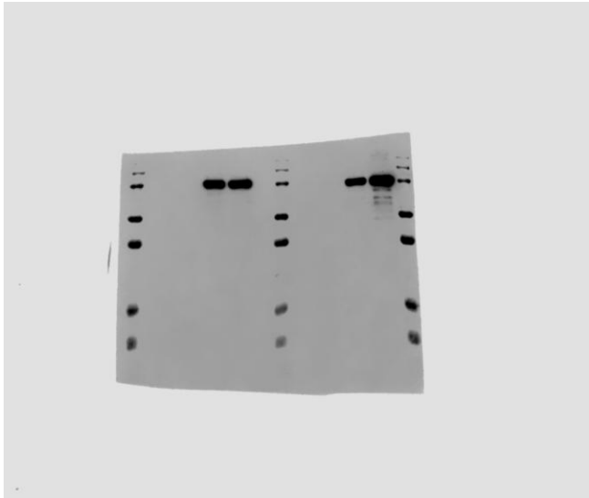
ALIX
