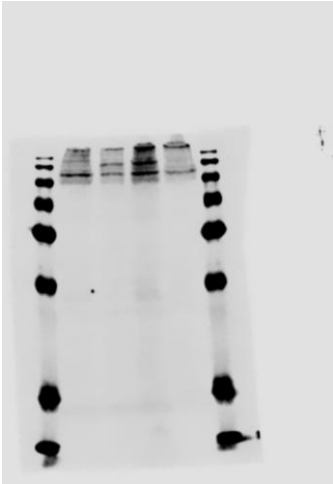
Alpha spectrin
