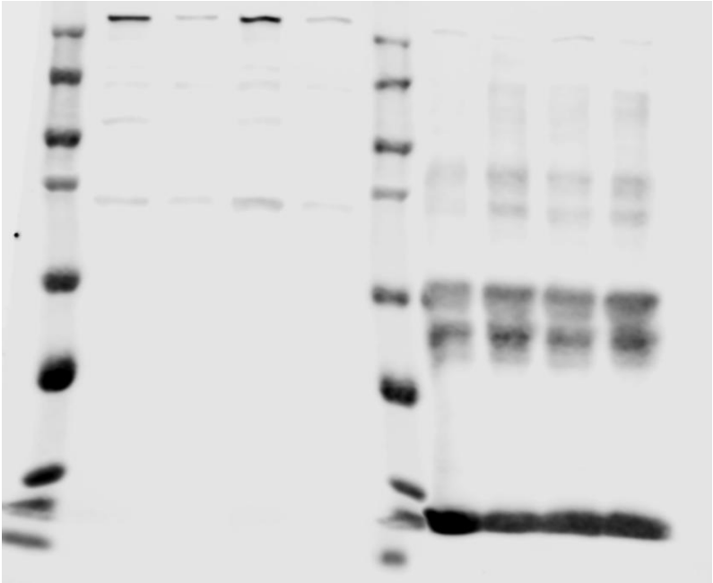
IgG
