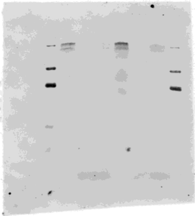
ALIX
