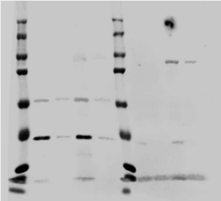
CHMP4B
