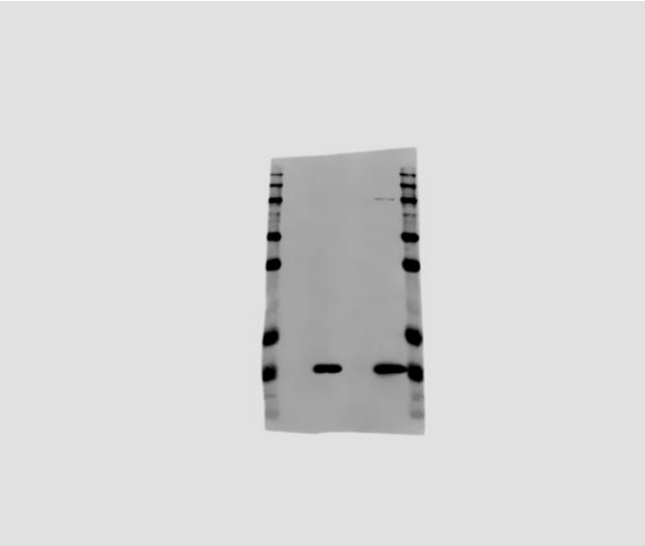
Caspase-2
