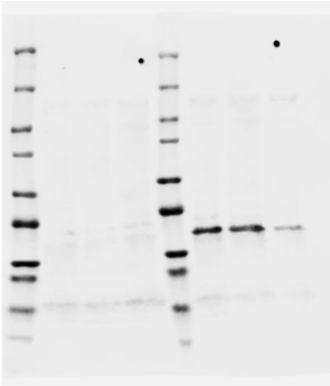
N-GSDMD
