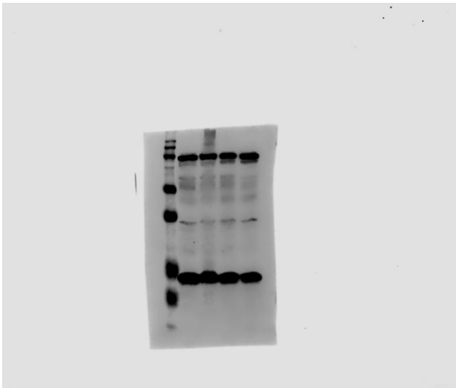
ALIX
