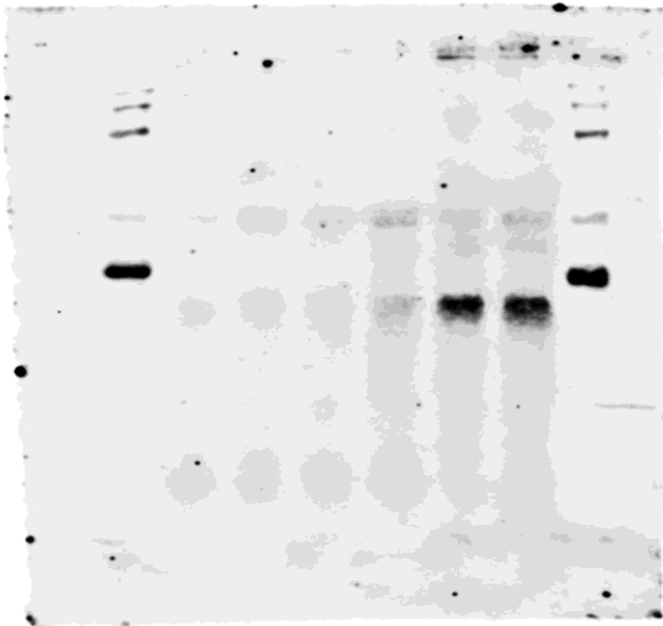
N-GSDMD
