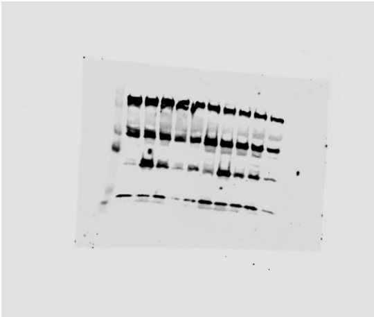
GSDMD
