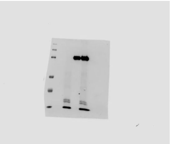
Caspase-4
