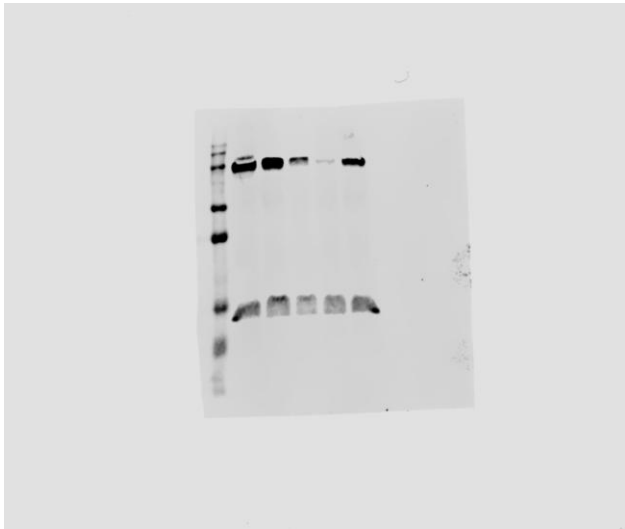
ALIX
