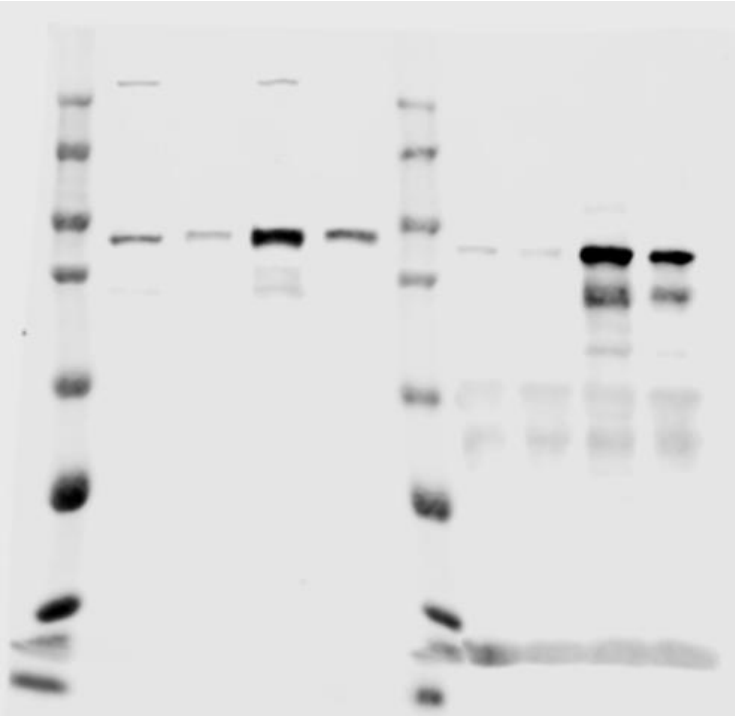
ALIX
