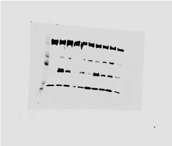
N-GSDMD
