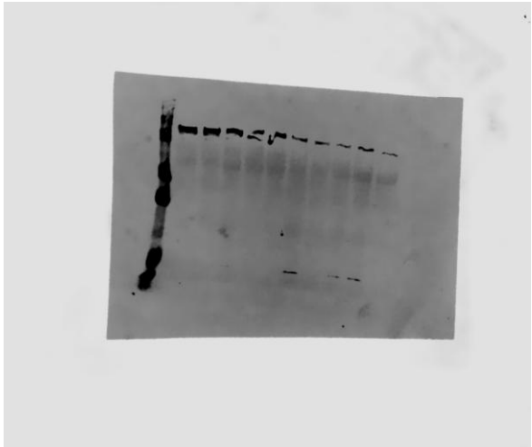
ALIX
