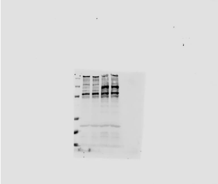
Alpha spectrin
