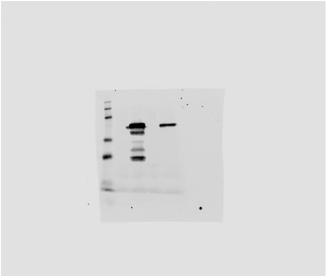
Flag-CAPN2
