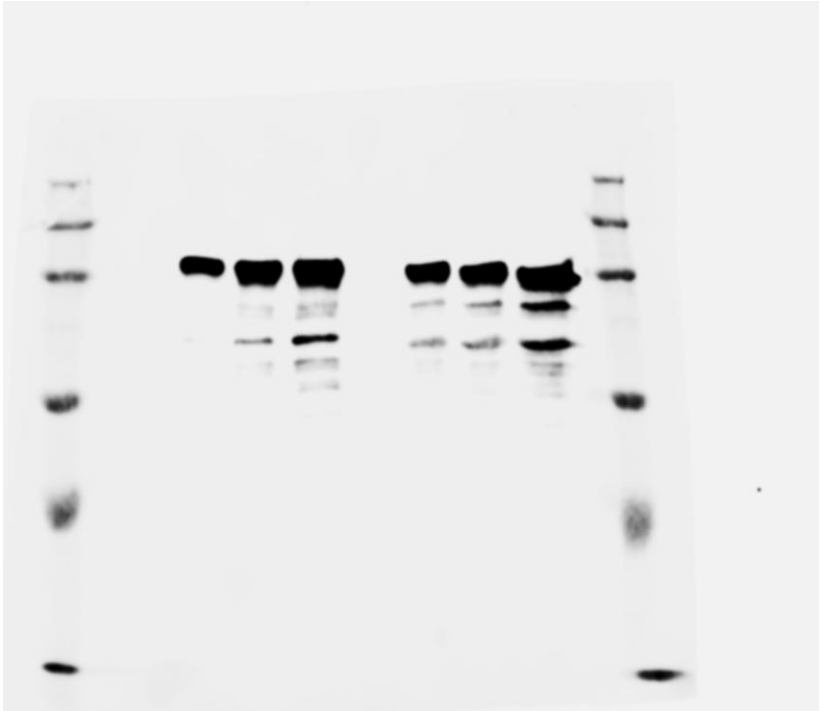
ALIX
