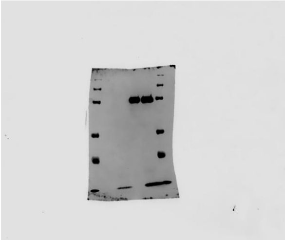
Caspase-3
