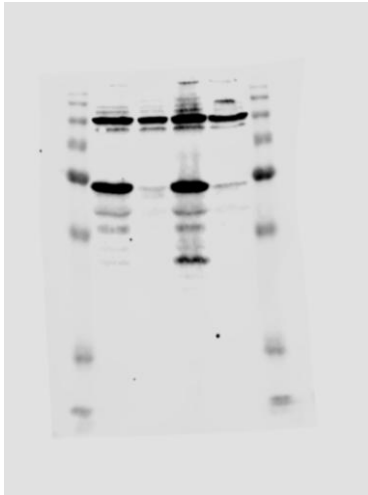
N-GSDMD
