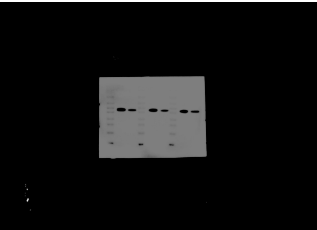
OCT4
