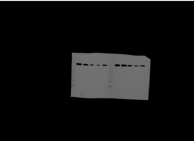
Drp 1
