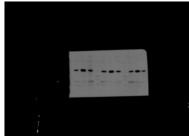
NANOG
