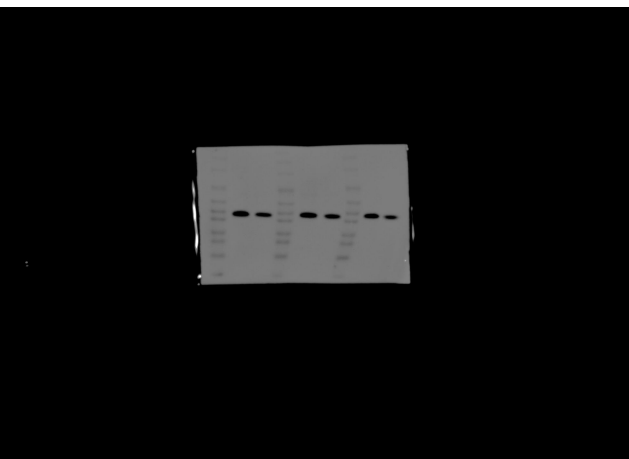
OCT4
