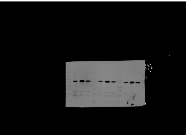
OCT4
