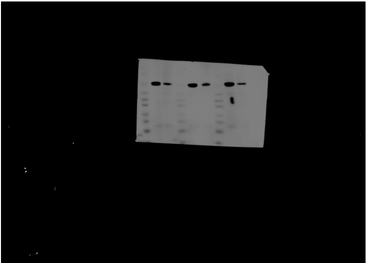
Drp 1
