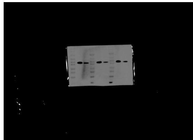
NANOG
