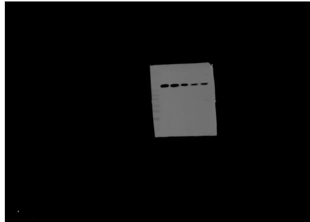
Drp 1
