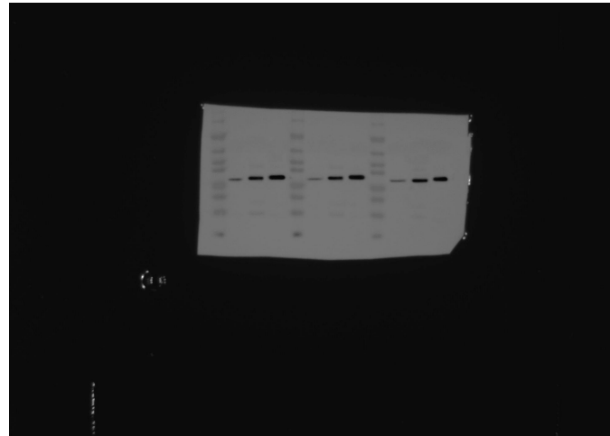
BAX
