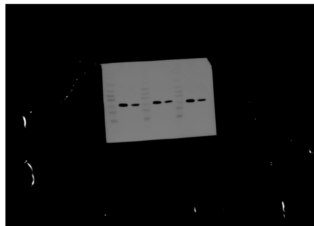
BAX
