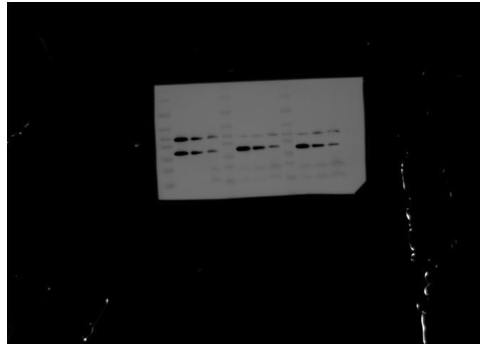
Bcl-2
