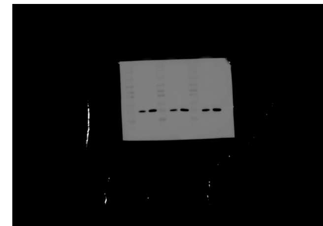
Bcl-2
