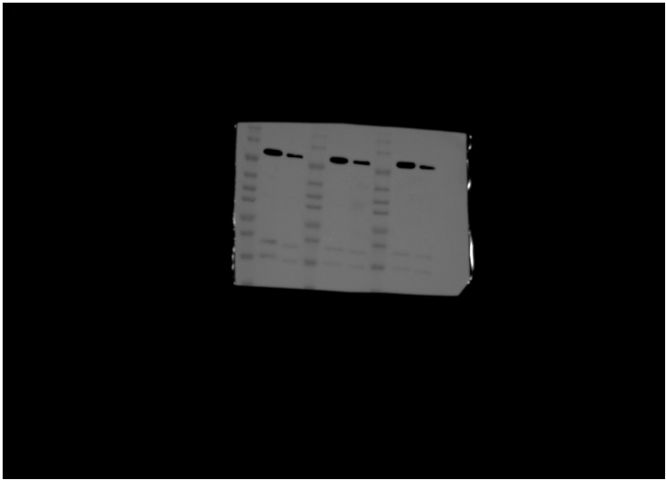
Drp 1
