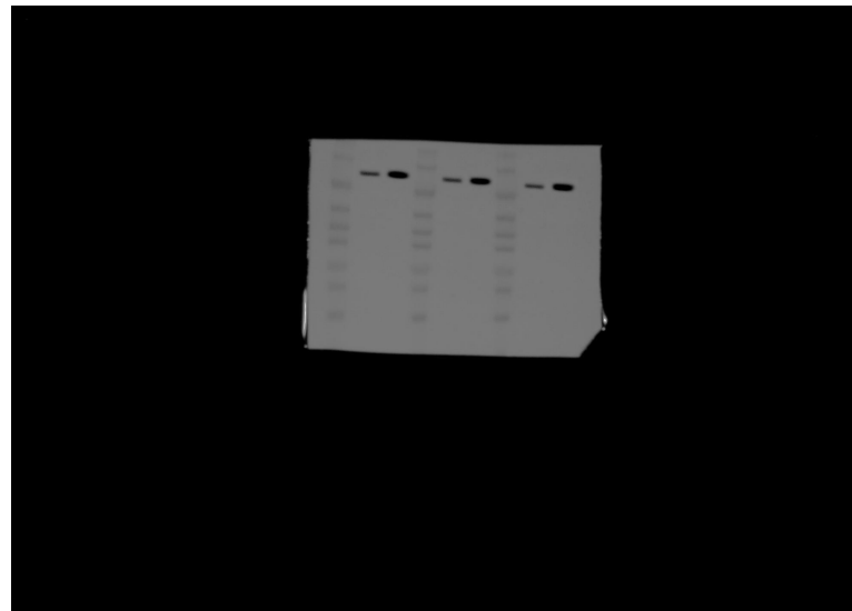
Drp 1
