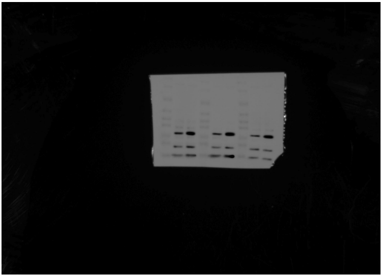
Bcl-2
