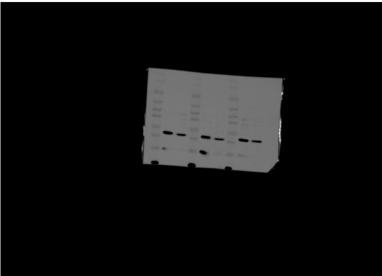
Bax
