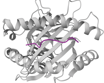
SEVGPEHSLAEY - HLA-B*44:03
