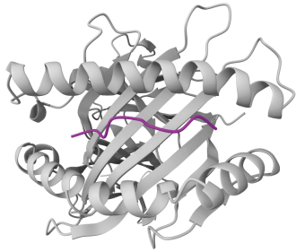
KTIQPRVEK - HLA-A*03:01
