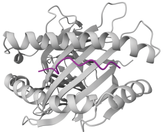
KTIQPRVEK - HLA-A*03:01
