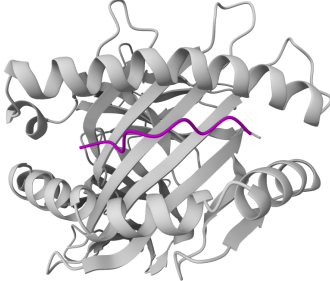
AEELAKNV - HLA-B*44:03
