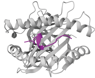
SEVGPEHSLAEY - HLA-B*44:03
